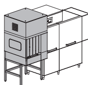
EVO/PRO DRA94MC 4,5 kW elektr. DRA99MC 9 kW elektr.
